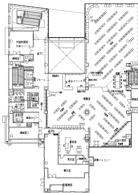
平面図
